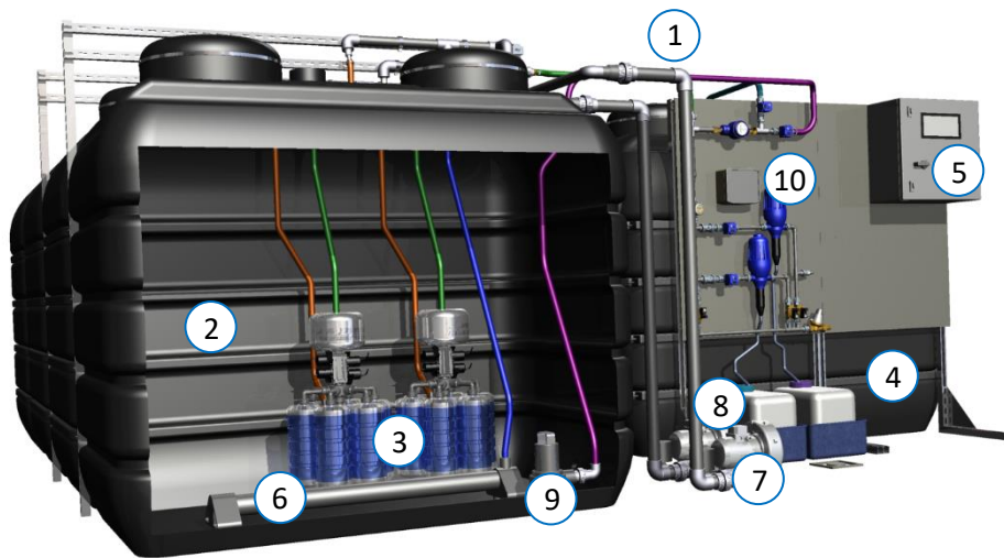
Abb 1.: Überblick: AQUALOOP Vorkonfektioniertes Grauwasser-Recycling Komplettsystem 21600 l/Tag Hinweis: Metallrack, Entwässerungsleitungen, Belüfterleitungen bauseits
