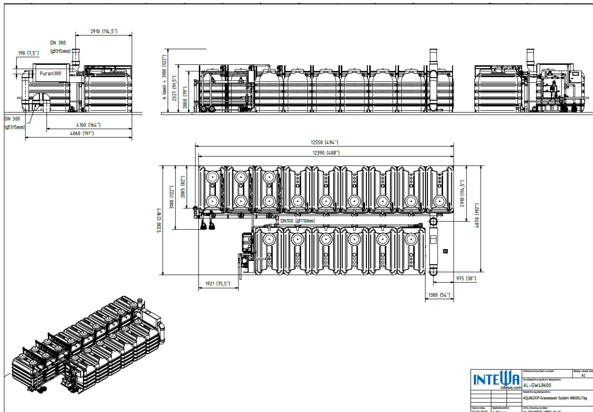
Abb. 2: Abmaße und Anschlüsse AQUALOOP AL-GW48600 I/d
