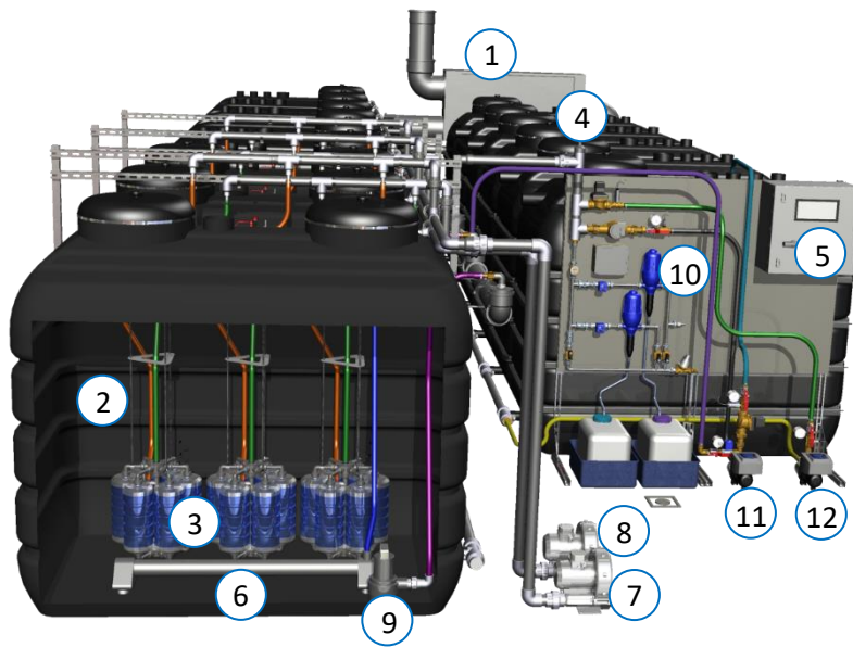
Abb1.: Überblick AQUALOOP Vorkonfektioniertes Grauwasser-Recycling Komplettsystem 48600 l/Tag Hinweis: Metallrack, Entwässerungsleitungen, Belüfterleitungen bauseits
