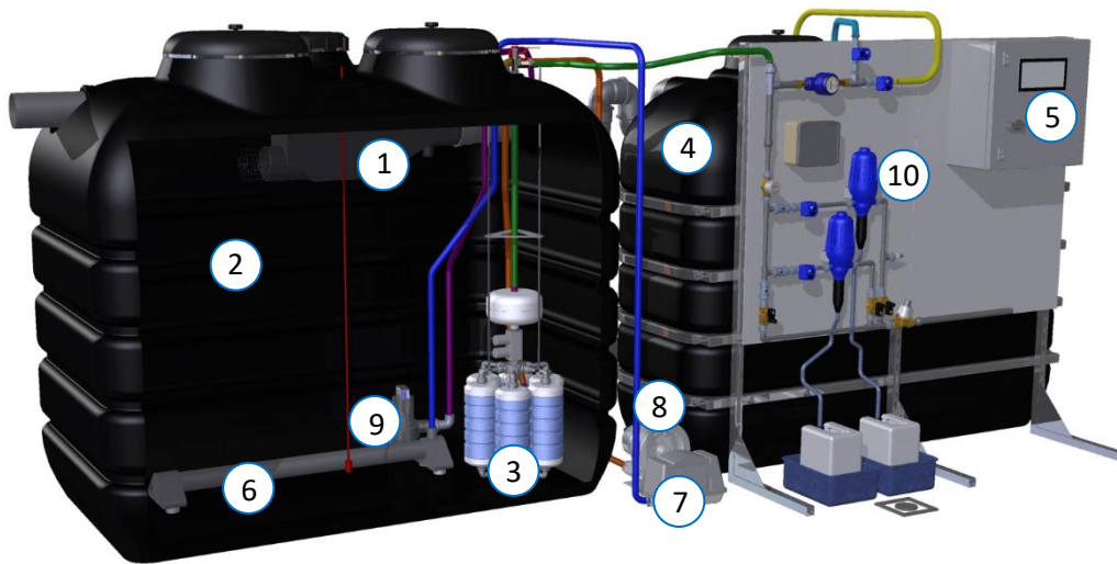
Abb 1.: Überblick AQUALOOP Vorkonfektioniertes Grauwasser-Recycling Komplettsystem 5400 l/Tag Hinweis: Metallrack, Entwässerungsleitungen, Belüfterleitungen bauseits
