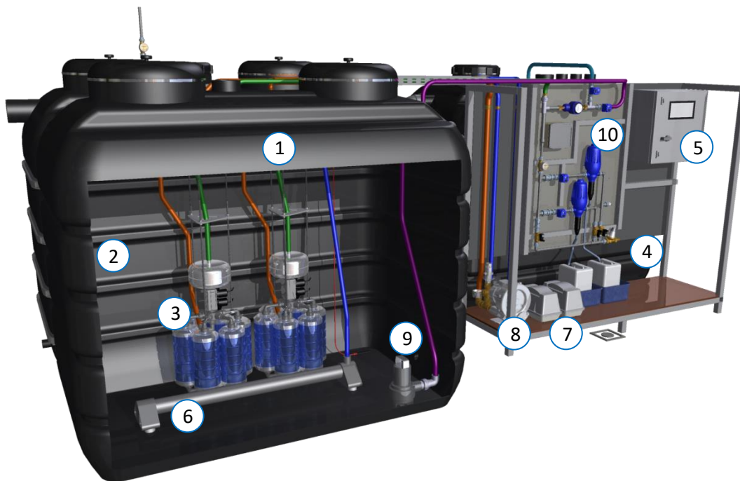
Abb 1: Überblick: AQUALOOP Vorkonfektioniertes Grauwasser-Recycling Komplettsystem 10800 l/Tag Hinweis: Metallrack, Entwässerungsleitungen, Belüfterleitungen bauseits
