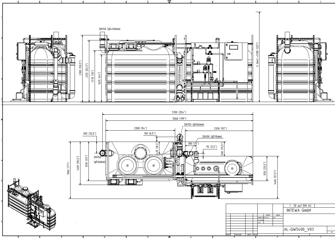
Abb. 2: Abmaße und Anschlüsse AQUALOOP AL-GW5400 I/Tag
