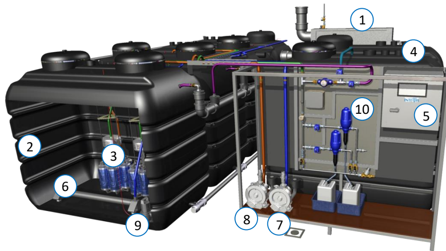
Abb 1.: Überblick: AQUALOOP Vorkonfektioniertes Grauwasser-Recycling Komplettsystem 21600 l/Tag Hinweis: Metallrack, Entwässerungsleitungen, Belüfterleitungen bauseits
