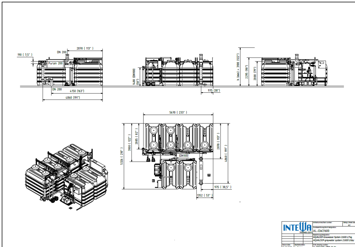
Abb.2: Abmaße und Anschlüsse AQUALOOP AL-GW21600 I/Tag
