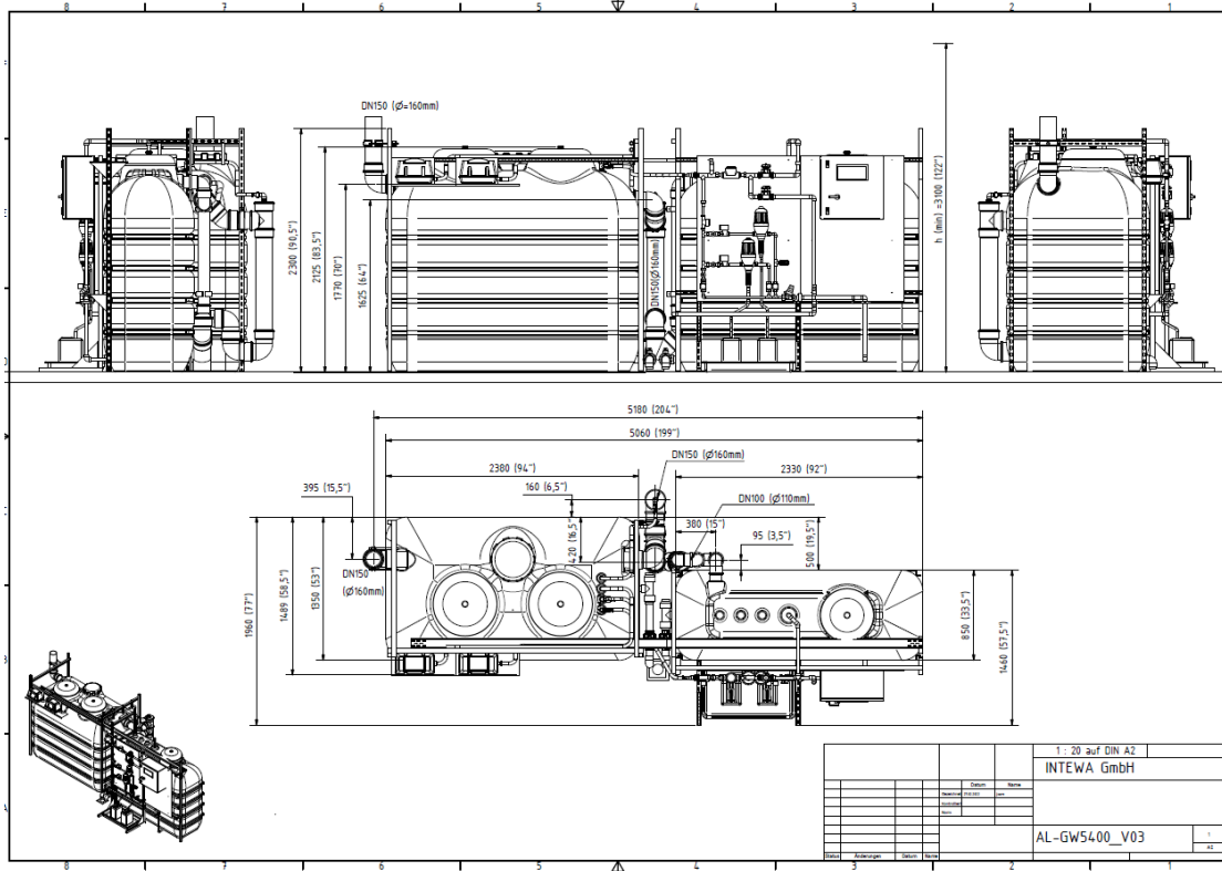
Abb. 2: Abmaße und Anschlüsse AQUALOOP AL-GW5400 I/Tag
